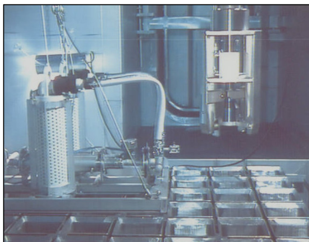
Televisuele inspectie in een desactivatiedok
